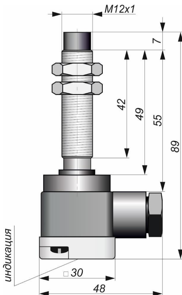
Габаритный чертеж
